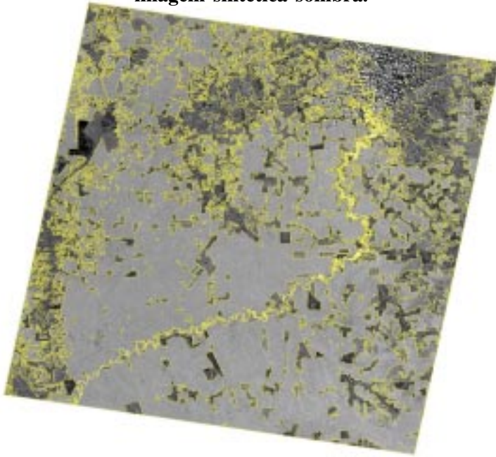
Fig. 3 As mesmas linhas de segmentação da figura 2 sobre a imagem colorida (R5 G4 B3) do sensor TM do satélite Landsat.
