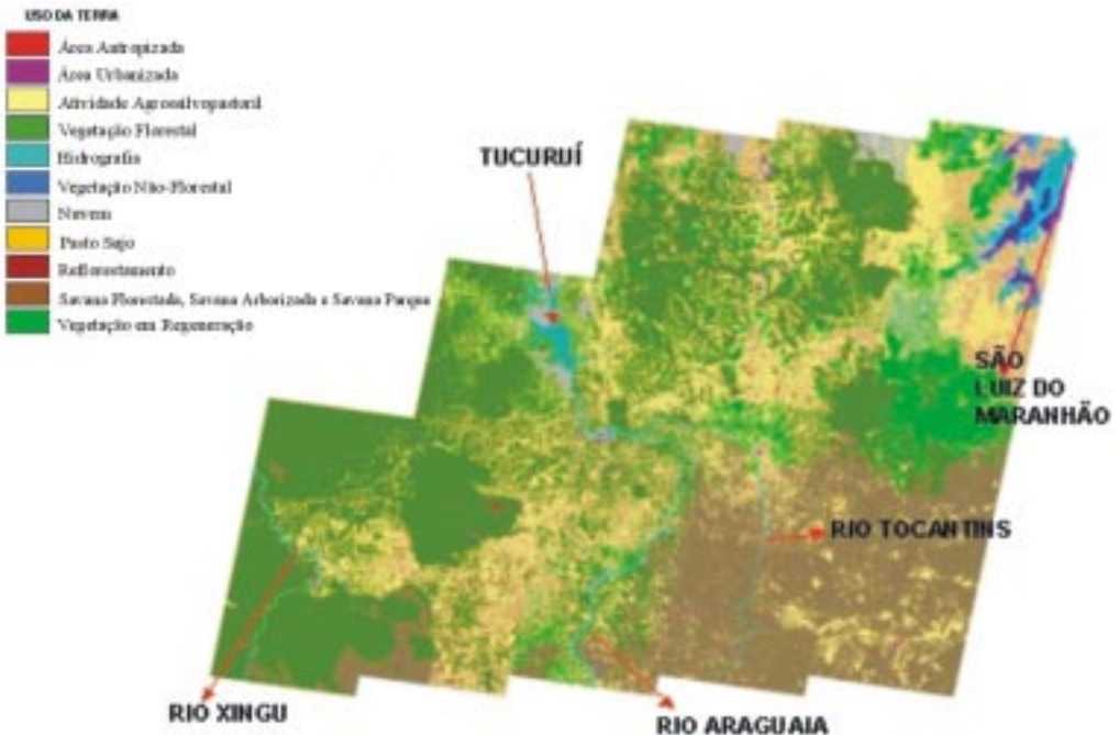
Fig. 10 Mapa da cobertura vegetal e do uso atual da terra da região de estudo.
