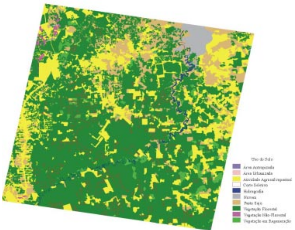
Fig. 9 Mapa final da imagem 223/62 do TM, obtido através do procedimento metodológico utilizado neste trabalho.
