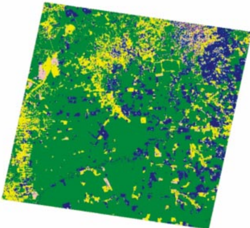
Fig. 7 Uma segunda classificação, apenas dentro das áreas desflorestadas, pode ser feita com o objetivo de mapear as outras classes de interesse (ex. pasto sujo, vegetação em regeneração etc.)
