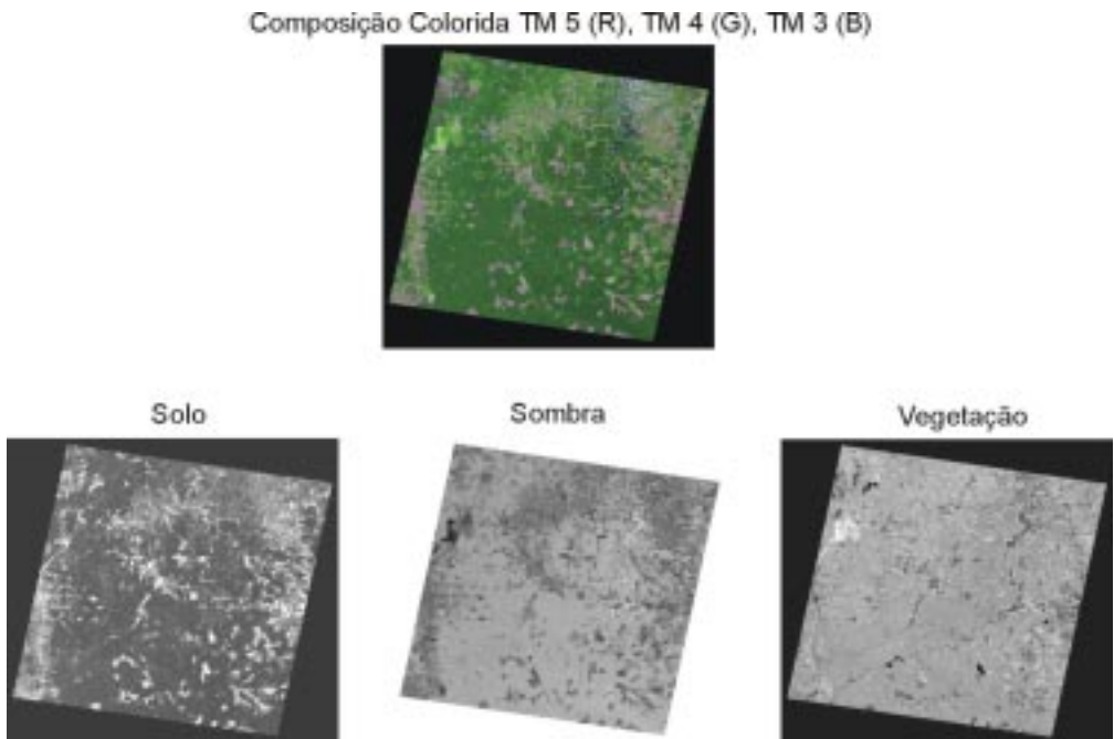
Fig. 1 Imagem Landsat TM (223/62) na composição colorida R5 G4 B3 (a) e as imagens sintéticas Solo (b), Sombra (c) e Vegetação (d) geradas a partir das bandas 3, 4 e 5 do TM, utilizando o modelo linear de mistura espectral
