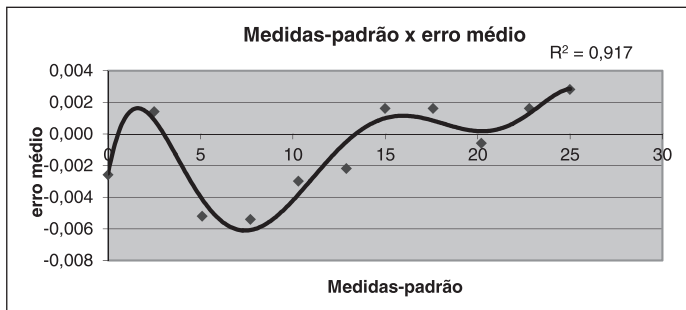
Figura 5 – Linha de tendência para as Medidas-padrão x Erro médio Fonte: próprio autor.
