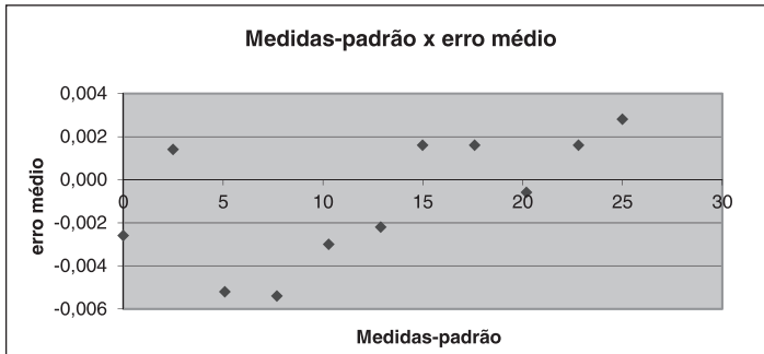
Figura 4 – Medidas-padrão x Erros das médio Fonte: próprio autor.
