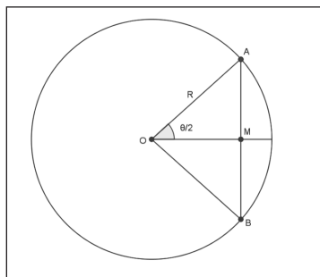
Figura 2 – Relação entre corda e seno. \theta/2 - metade do ângulo central AÔB; R - raio da circunferência; AB - corda; AM - meia corda.
